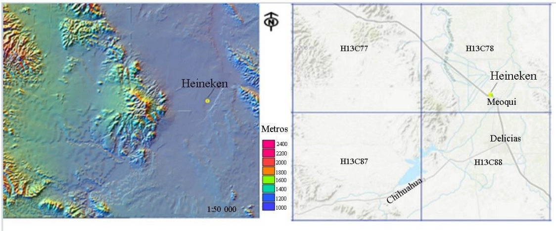
Figura 5. Modelo digital de elevación. Área de influencia planta Cuauhtémoc-Moctezuma Meoqui, Chihuahua. Fuente: elaboración propia con datos del INEGI (2023). Continuo de elevaciones mexicano.
