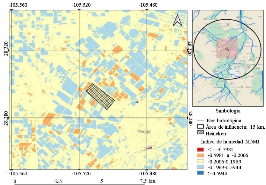
Figura 9. Índice de humedad. Zona de influencia planta Cuauhtémoc-Moctezuma Meoqui. Fuente: elaboración propia con datos de European Space Agency.
