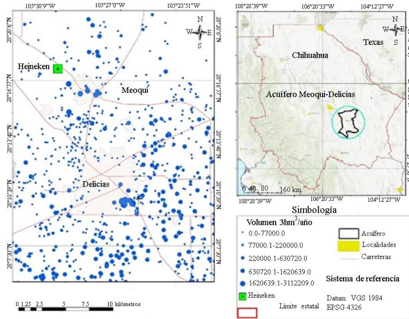
Figura 1. Ubicación planta Cuauhtémoc-Moctezuma Meoqui y concesiones para extracción de agua subterránea según volumen \text{hm}^3/\text{año} en zona de estudio. Fuente: elaboración propia. Registro público de derechos de propiedad, (Conagua, 2023).
