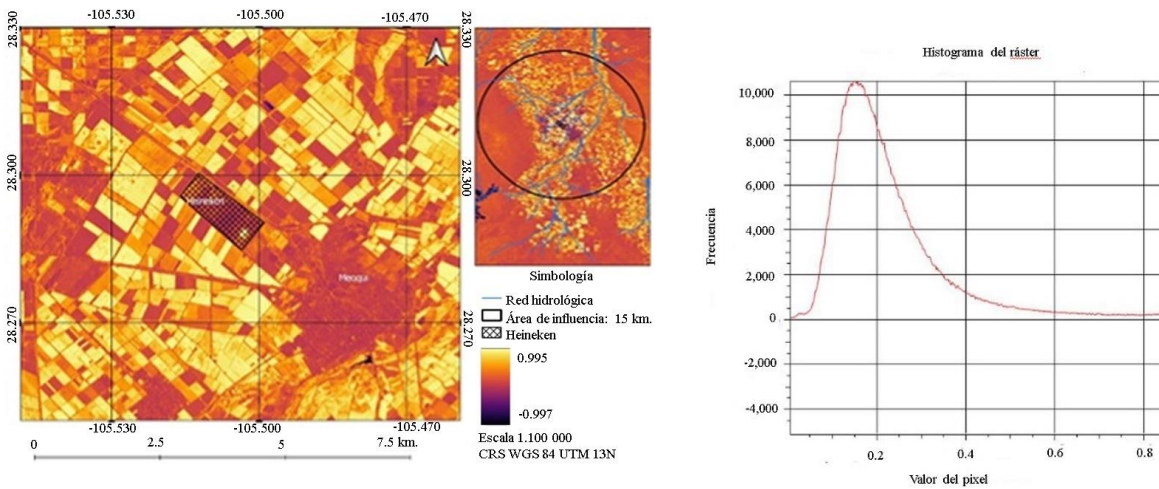
Figura 8. Índice de vegetación NDVI. Zona de influencia planta Cuauhtémoc-Moctezuma Meoqui. Fuente: elaboración propia con datos de European Space Agency.
