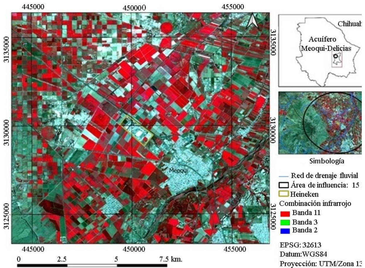
Figura 7. Combinación de color infrarrojo. Zona de influencia planta Cuauhtémoc-Moctezuma Meoqui. Fuente: elaboración propia con datos de European Space Agency.
