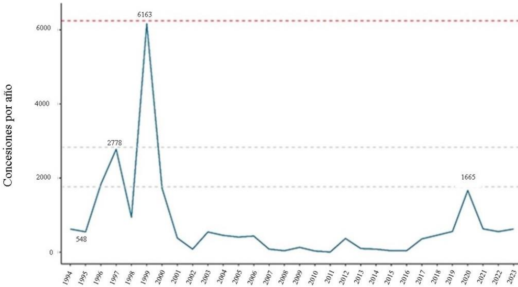
Figura 4. Evolución temporal de las concesiones para extracción de agua subterránea en Chihuahua. 1993-2023. Fuente: elaboración propia con datos de Repda (Conagua, 2023).
