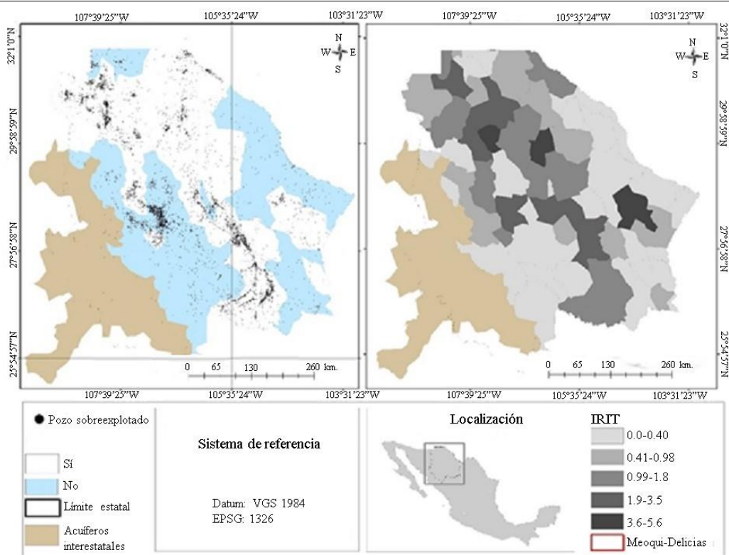
Figura 2. Índice Relativo de Intensidad Territorial (IRIT, 2023). Distribución de concesiones para extracción de agua subterránea (pozos) de Chihuahua y clasificación de acuíferos según estatus de sobreexplotación. Fuente: datos del Registro público de derechos de propiedad. (Conagua, 2023).
