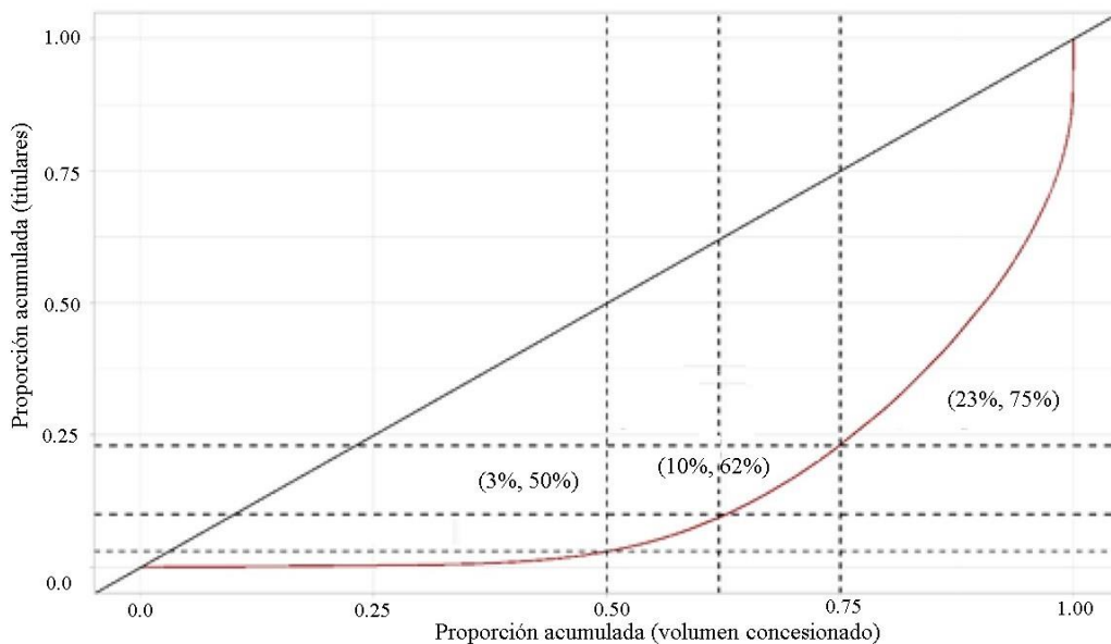
Figura 3. Curva de Lorenz. Distribución del volumen concesionado en acuíferos de Chihuahua, 2023. Fuente: elaboración propia con datos de REPGA (Conagua, 2023).
