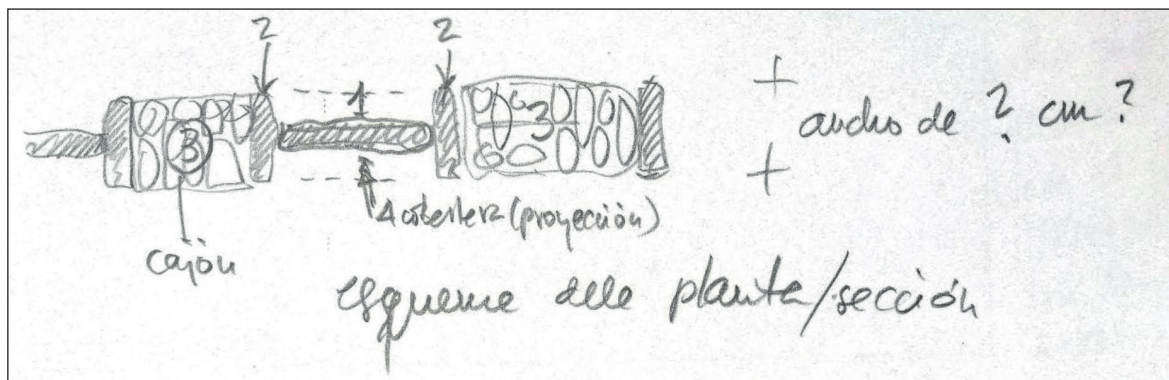
Figura 1. Esquema de pared de piedra seca. Dibujo de corrección/ampliación/discusión a uno de los de mi tesis doctoral. Dibujo de JGB.
