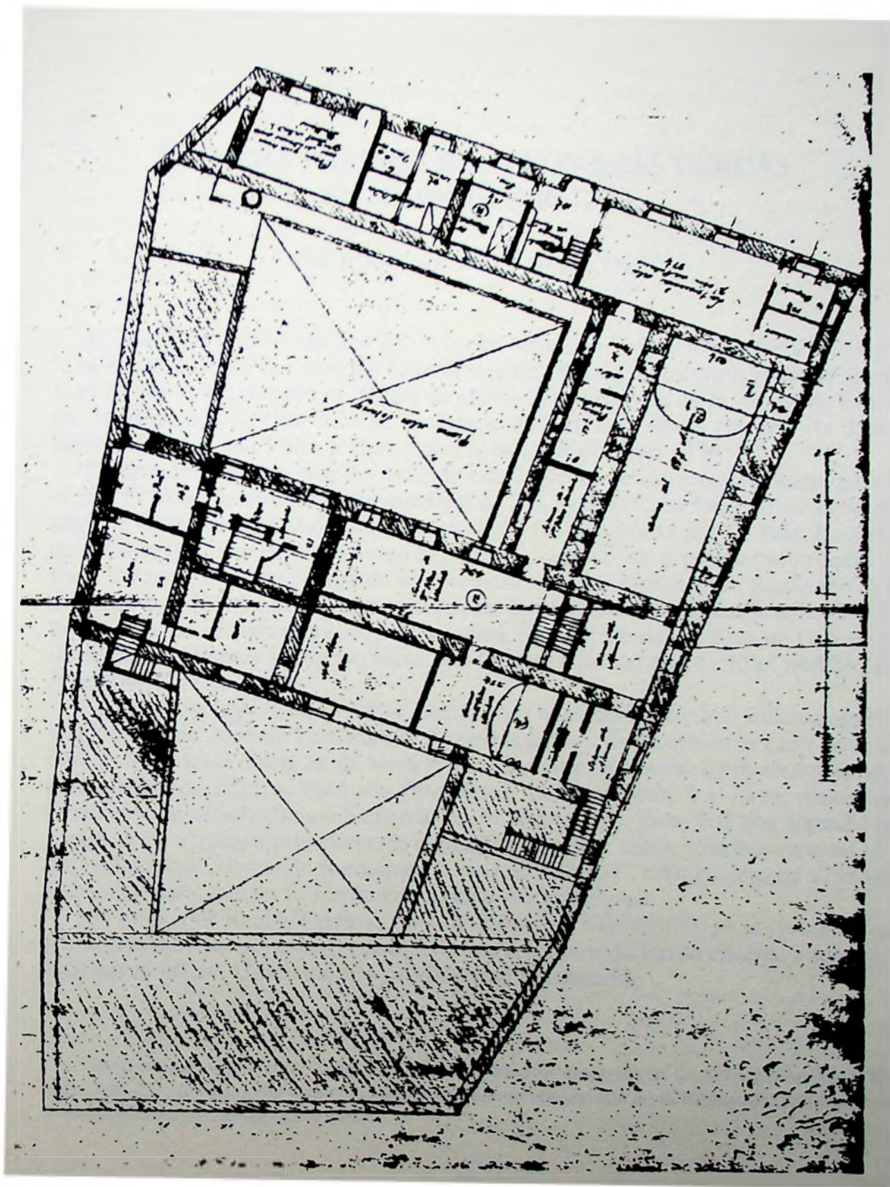
Fig. 3. Madrid. "Casa de Rebeque": sótano.
