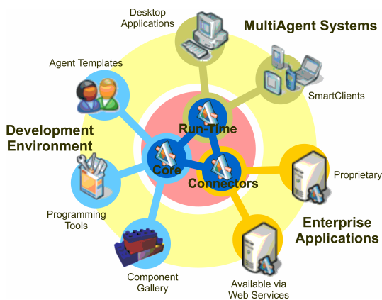
Figura 1 Arquitectura CAPNET.
