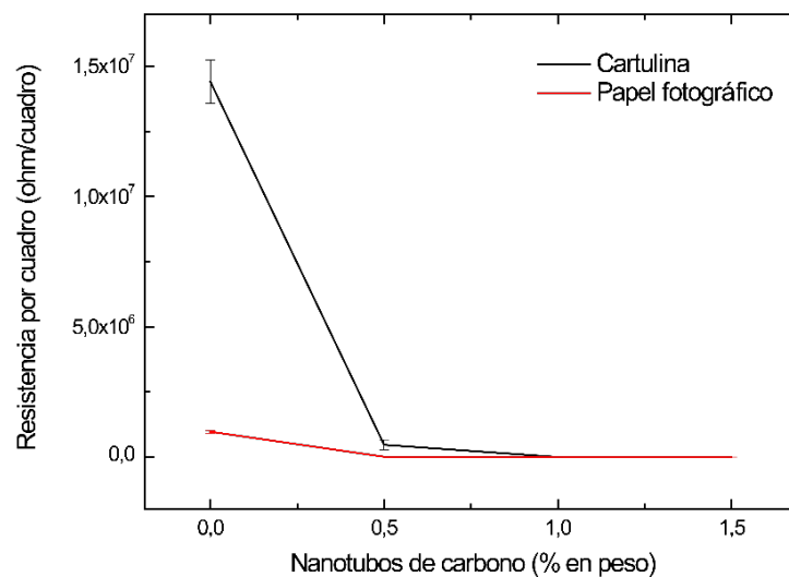
Figura 3. Dependencia de la resistencia por cuadra de la tinta con el % en peso de los NTC.
