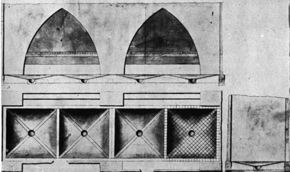
LÁMINA 2.—Planta, perfiles y alzado de las naves del extremo sur de las Atarazanas Reales de Sevilla (Servicio Geográfico del Ejército. Ministerio del Ejército. Madrid).
