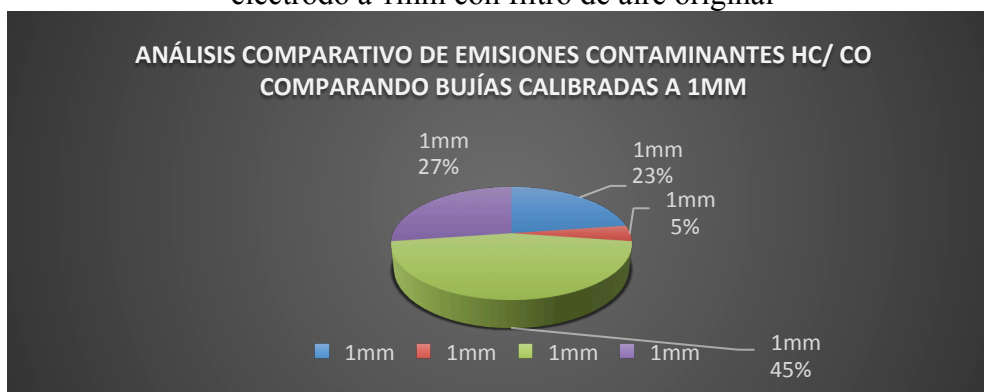
Figura 9. Análisis de Gases a 2500rpm combustible 92 octanos variable bujía calibración electrodo a 1mm con filtro de aire original
