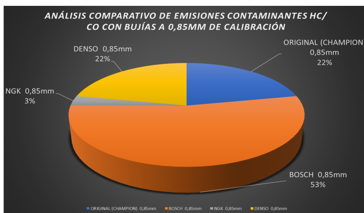
Figura 11. Análisis de Gases a 700rpm combustible 87 octanos variable bujía calibración electrodo a 0.85mm con filtro de aire original
