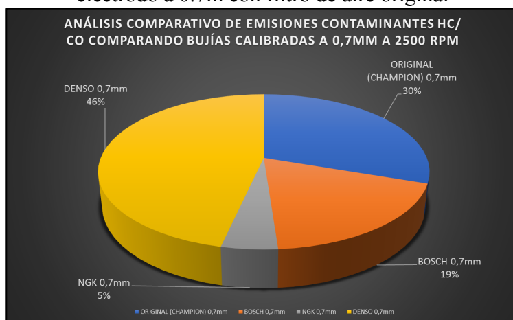
Figura 13. Análisis de Gases a 2500rpm combustible 87 octanos variable bujía calibración electrodo a 0.7m con filtro de aire original
