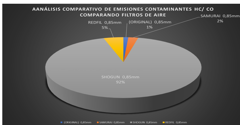
Figura 12. Análisis de Gases a 700rpm combustible 87 octanos variable filtros de aire con bujía NGK electrodo a 0,85mm
