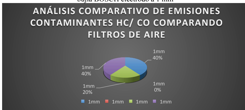
Figura 8. Análisis de Gases a 700rpm combustible 92 octanos variable filtros de aire con bujía BOSCH electrodo a 1 mm
