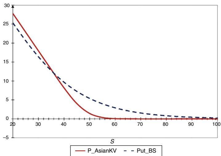
Figura 2. Comparación entre precios de opciones asiáticas de venta con el modelo de Kemna y Vorst (1990) y con el modelo de Black y Scholes (1973) . Fuente: elaboración propia.
