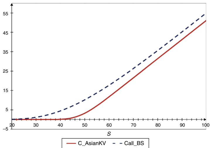
Figura 1. Comparación entre precios de opciones asiáticas de compra obtenidos con el modelo de Kemna y Vorst (1990) y con el modelo de Black y Scholes (1973) . Fuente: elaboración propia.
