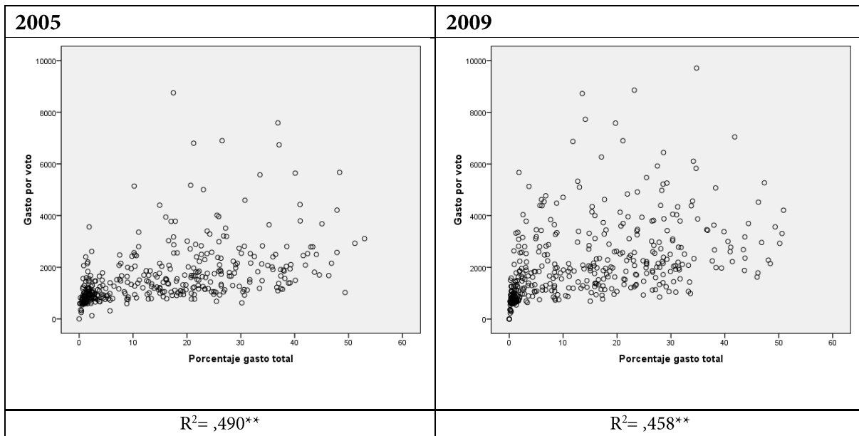
Diagrama de dispersión entre PGT y GPV
