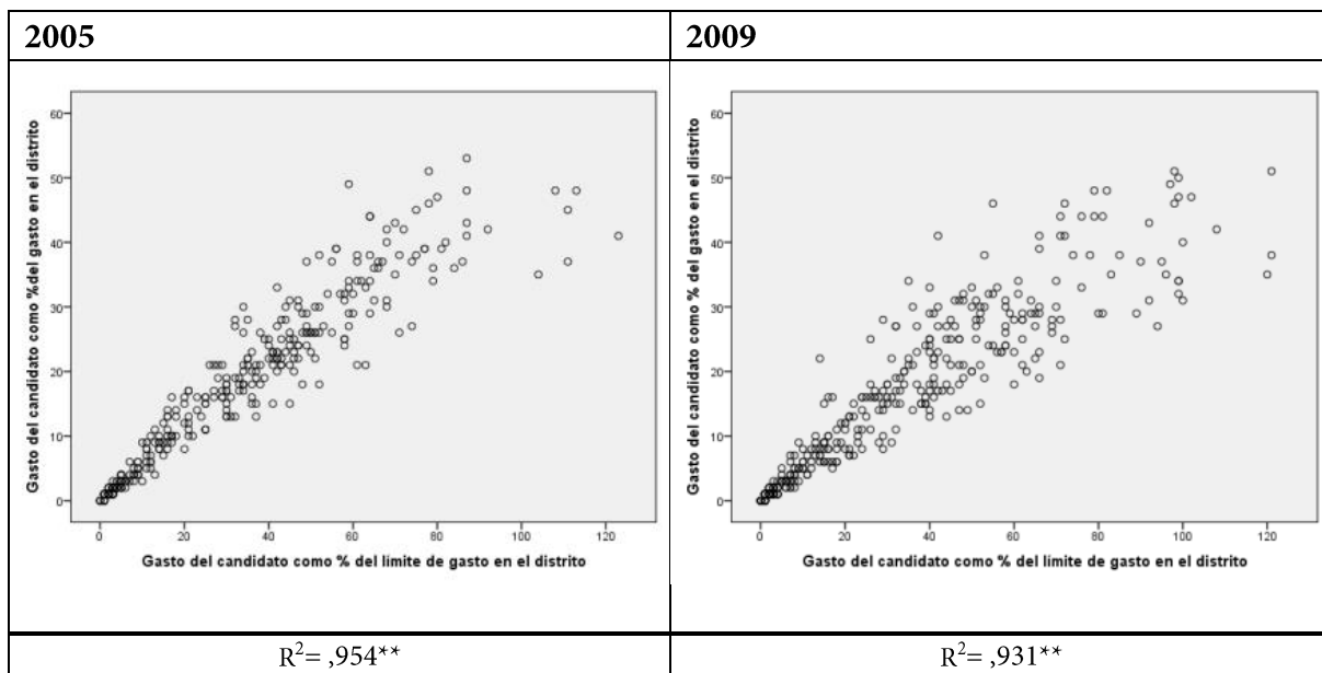
Diagrama de dispersión entre PorLG y PGT
