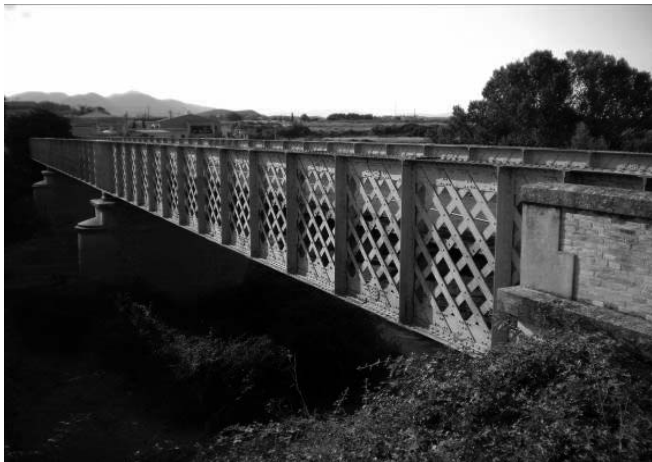
Elementos del patrimonio de las carreteras en la Región de Murcia de finales del siglo XIX: puente metálico de Cehegín en la carretera de tercer orden de Murcia a La Puebla de Don Fadrique Fuente: Fotos del autor.
